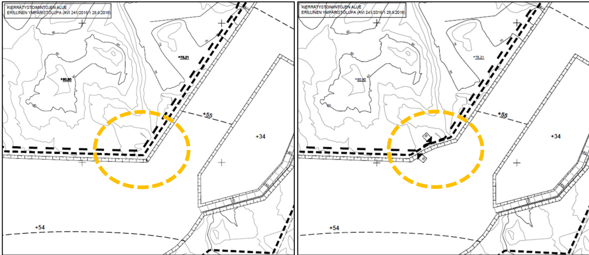
Kuvat 1 ja 2. Ote luvan TUUDno-2019-645 mukaisesta lopputilannekuvasta vasemmalla ja ote päivitetyistä suunnitelmapiirustuksesta oikealla (piirustus S2A). Kuviin on ympyröity alue, jossa luvan mukaisesta ottoalueesta on poikettu (lisätty jälkikäteen).
