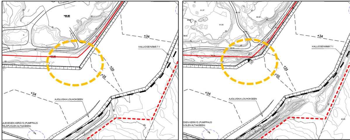
Kuvat 5 ja 6. Ote luvan ESAVI/41056/2022 vaiheen 2 mukaisesta lopputilannekuvasta vasemmalla ja ote päivitetystä suunnitelmapiirustuksesta oikealla (piirustus S3B). Kuviin on ympyröity alue, jossa luvan mukaisesta ottoalueesta on poikettu (lisätty jälkikäteen).
