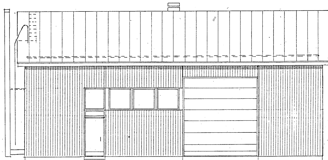
JULKISIVU ETELÄÄN 1 : 100
