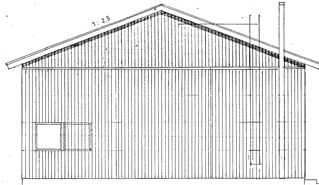
PÄÄTY LÄNTEEN 1 : 100
